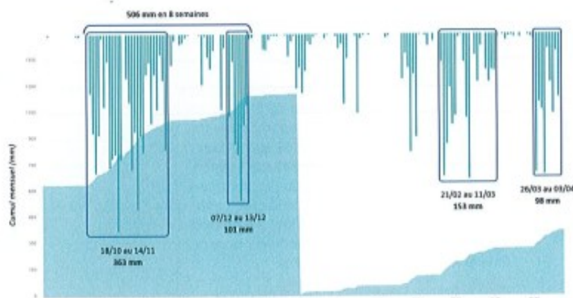
Pluviométrie sur le bassin de la Charente
